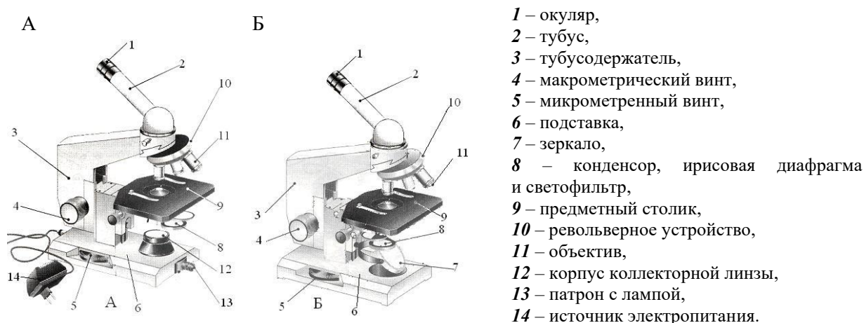
Рисунок 1 – Строение электронного (А) и светового (Б) микроскопов
