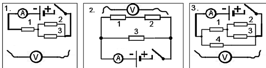
Рисунок 4.6 – Варианты электрических схем со смешанным соединением проводников
