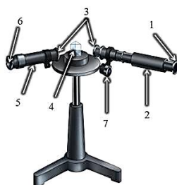
Рисунок 9.2– Устройство спектрографа двухтрубного
